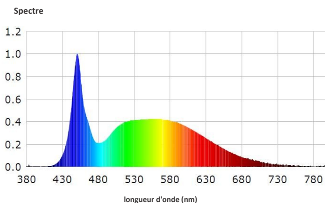
Courbe Photométrique
